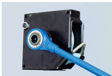
Sexkant på axeln för kombinerad stång med spärrnyckel.
