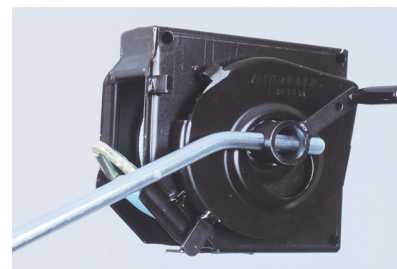
Bandet spänns med spännstång av seghärdat stål.
